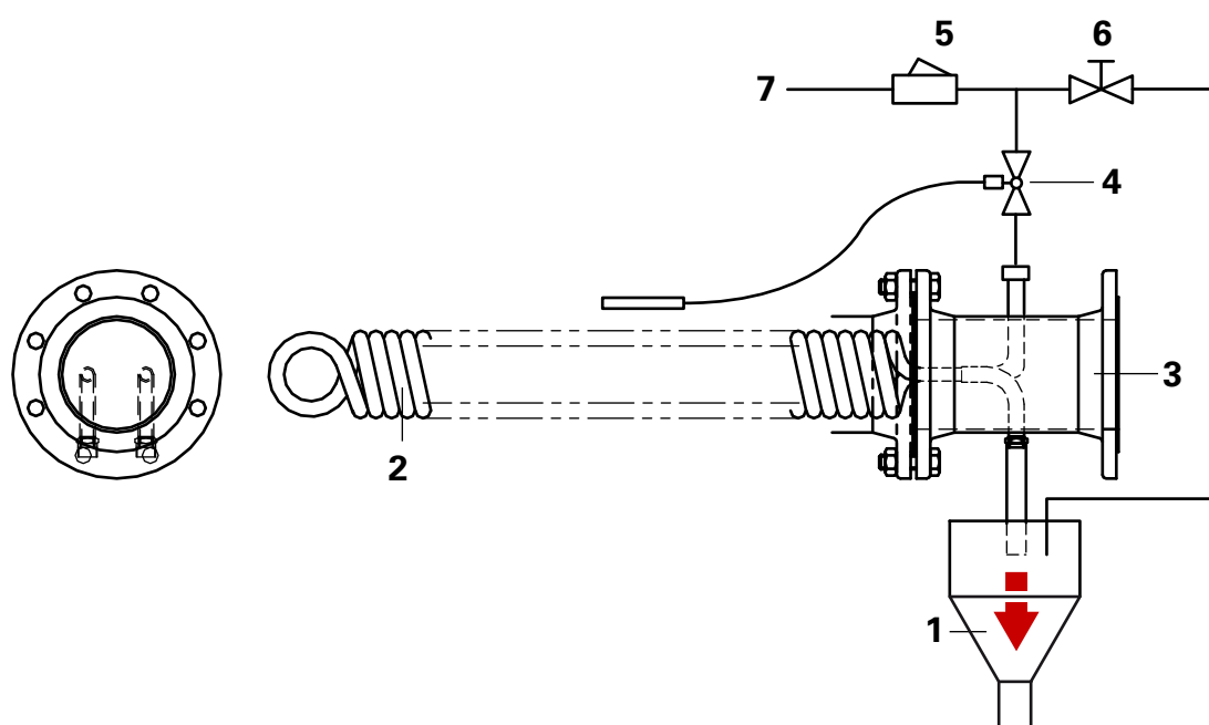
avb. 8 Termisk utløpsikring
