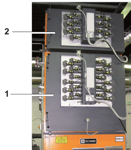
avb. 11 Fyringsanlegg med varmtvannskjele og ettervarmeveksler
