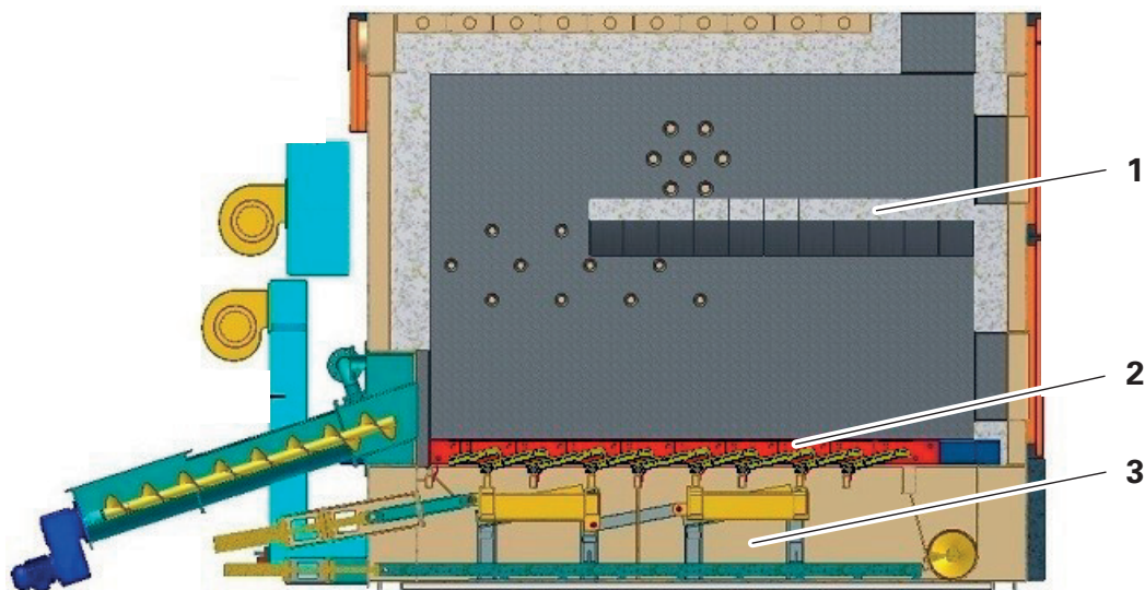
Fig. 14 Nettoyage
