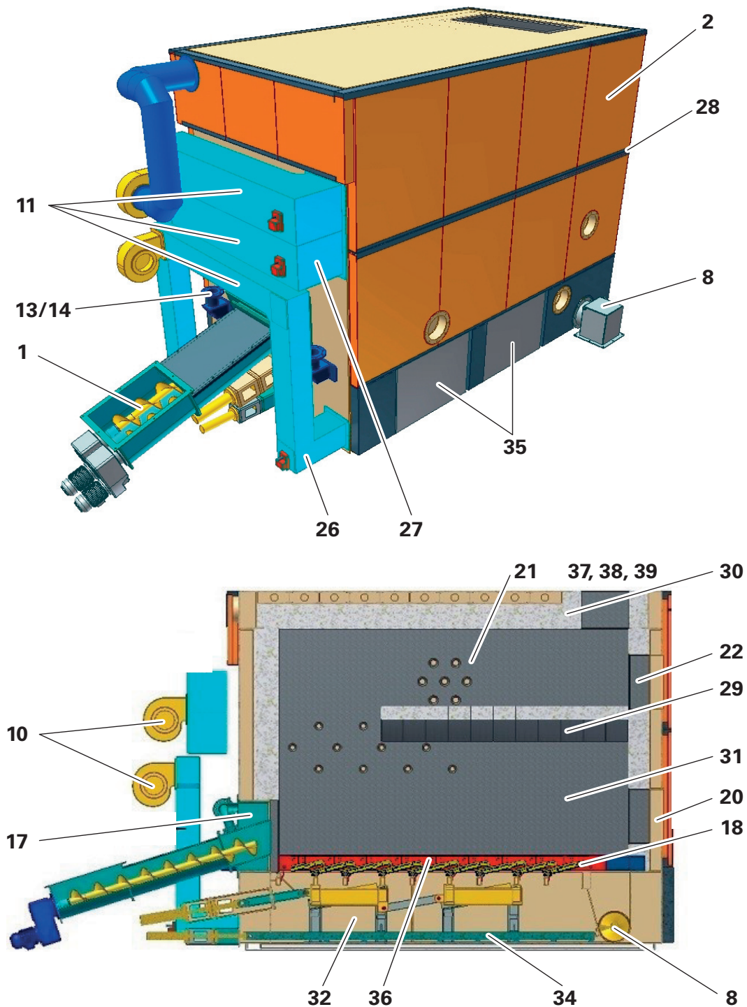
Fig. 5 Construction de la chaudière à grille mobile
