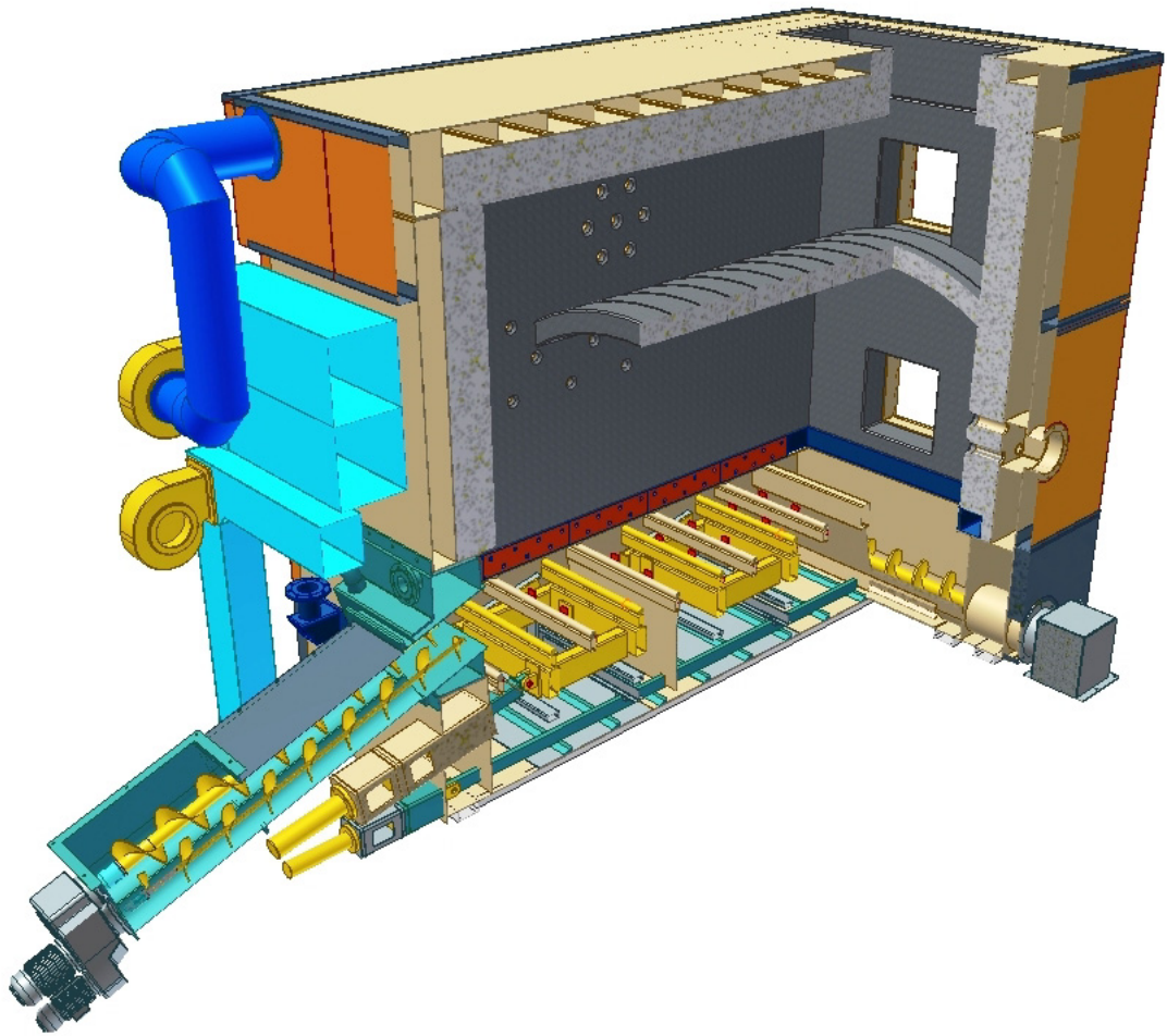
Fig. 3 Coupe de la chaudière à grille mobile
