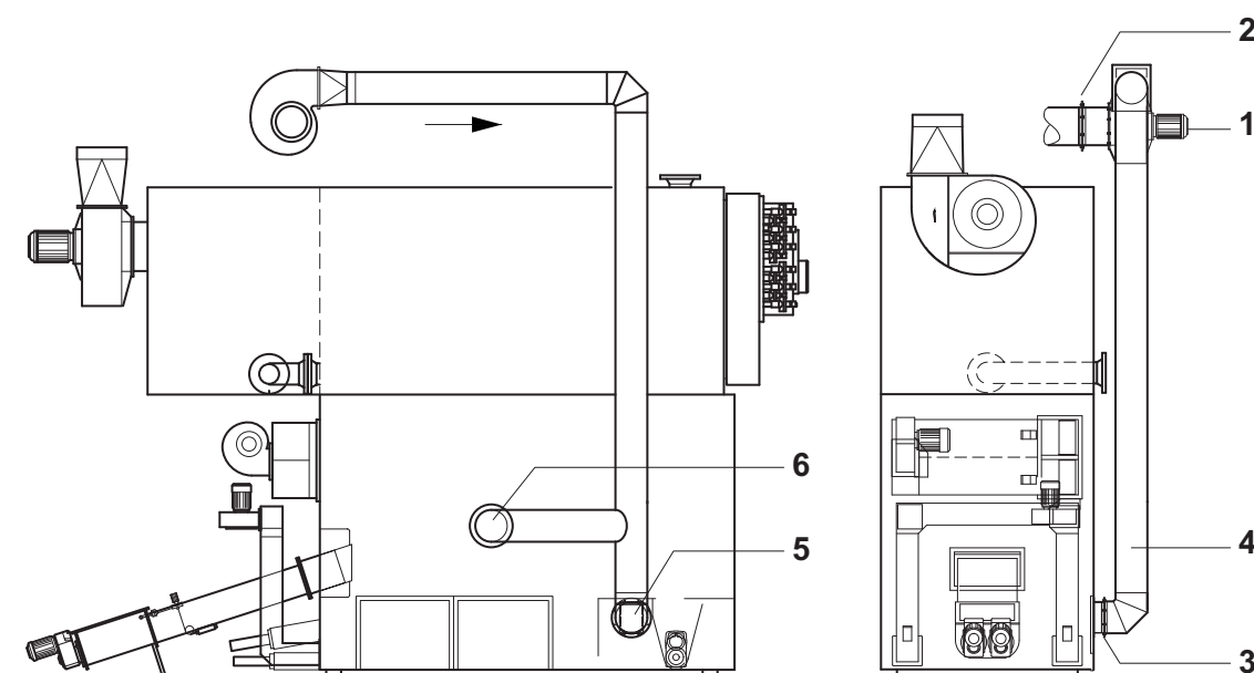
Fig. 8 Recirculation des fumées (exemple illustré)
