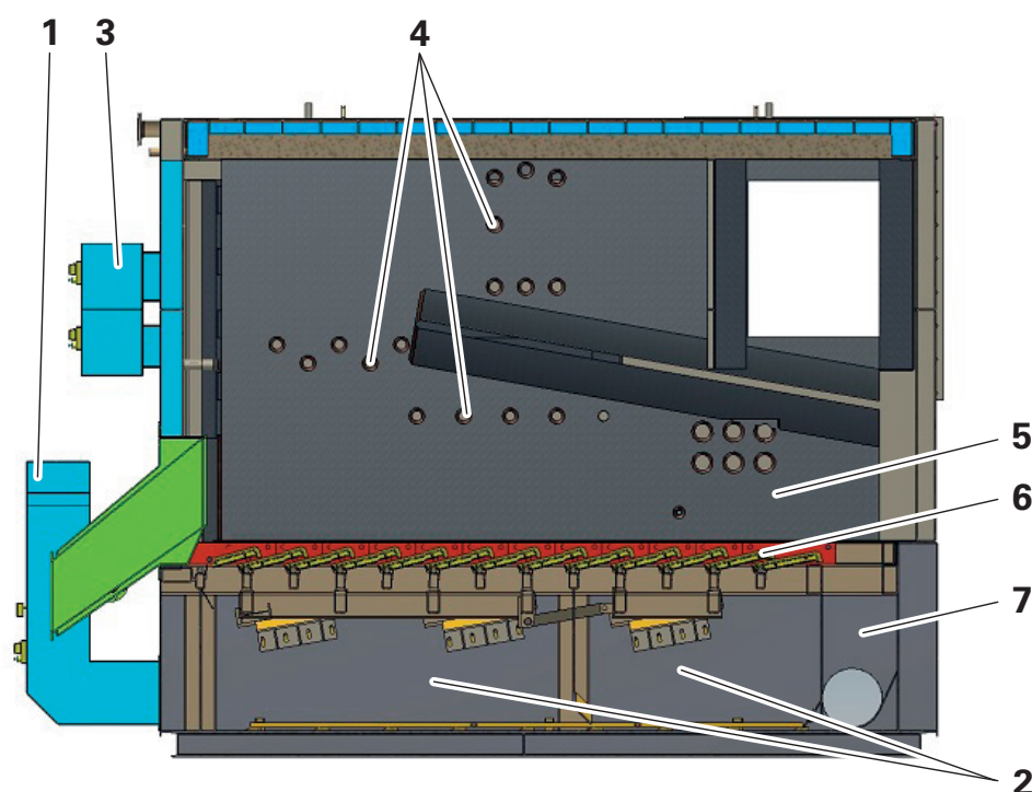
Fig. 4 Structure fondamentale
